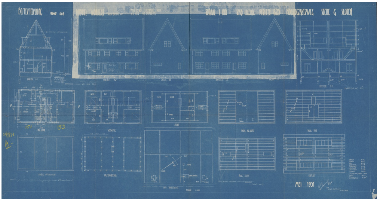
Bouwtekening woonhuis Noorderakerweg 151/153, mei 1931 (Familiearchief M.W.A.G. Wielart-Berendsen)
